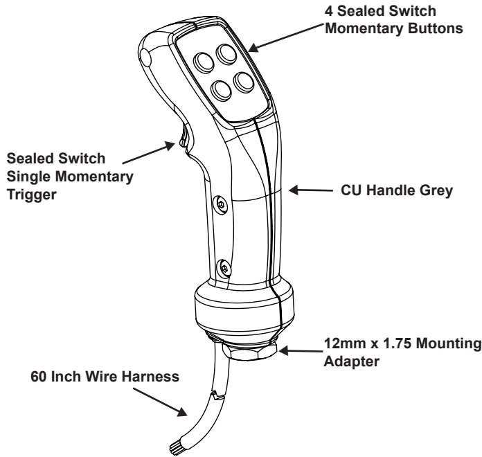
CU Example 3
