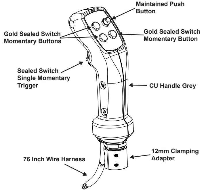
CU Example 4
