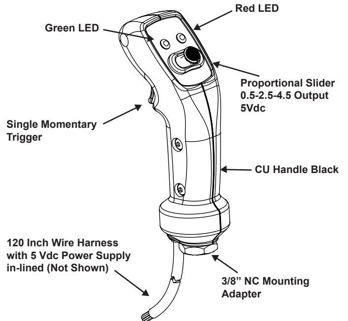
CU Example 4
